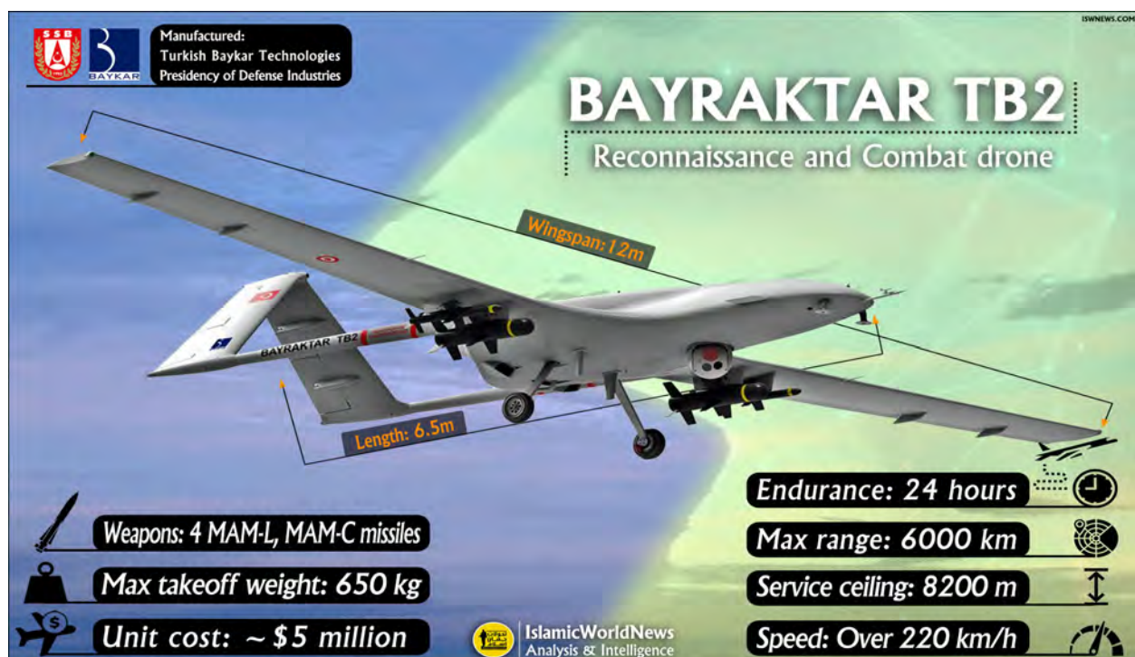
Abbildung 7: Die „BAYRAKTAR TB2“, der türkische „Gamechanger“ in den Konflikten in den Kurdengebieten, Syrien, Libyen und in Karabach. 56
